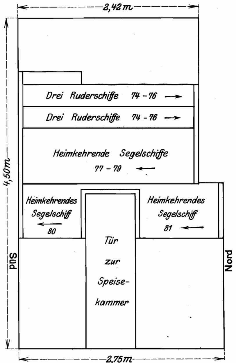
Korridor II: Westwand
